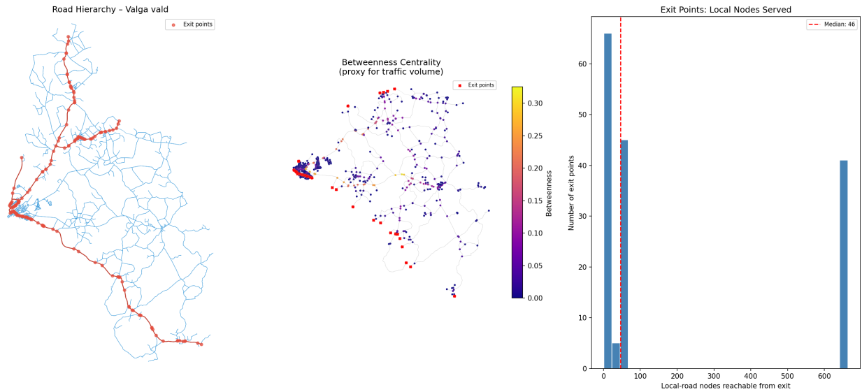
Joonis 1. Valga vald maateede võrgustiku ülevaade.
